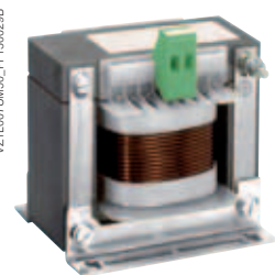
VZ1L0●●●UM●0
