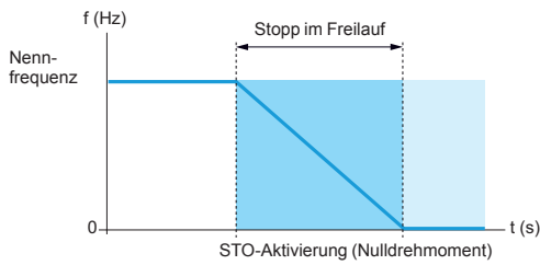
Aktivierung der Sicherheitsfunktion STO
