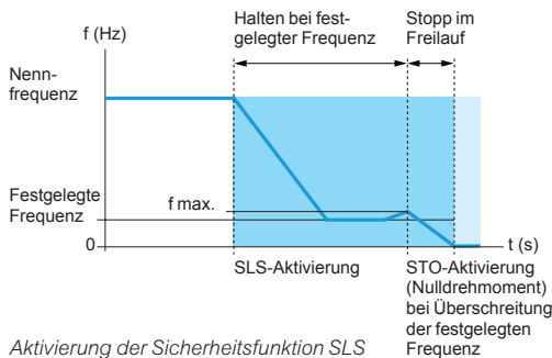
Aktivierung der Sicherheitsfunktion SLS
