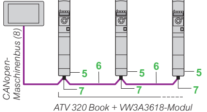
Beispiel für den Anschluss an den CANopen-Maschinenbus über den SUB-D-Steckverbinder
