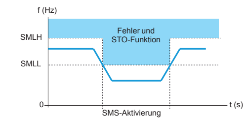
Aktivierung der Sicherheitsfunktion SMS
