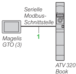
Beispiel für den Anschluss eines Umrichters Altivar 320 in Buchbauform und eines HMI-Terminals Magelis GTO über die serielle Modbus-Schnittstelle
