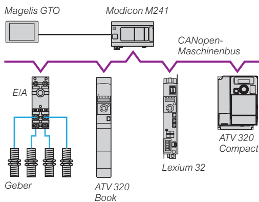
Beispielkonfiguration mit CANopen-Maschinenbus
