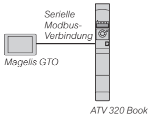
Beispielkonfiguration mit serieller Modbus-Verbindung
