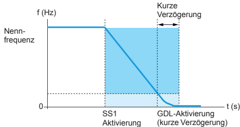
Aktivierung der Sicherheitsfunktion GDL (Beispiel für Stopp-Typ: SS1)
