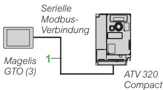
Beispiel für den Anschluss eines Umrichters Altivar 320 in Kompaktbauform und eines HMI-Terminals Magelis GTO über die serielle Modbus-Schnittstelle
