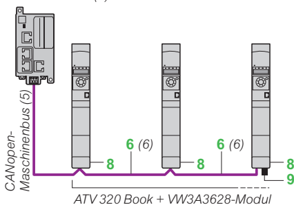
Beispiel für den Anschluss an den CANopen-Maschinenbus über Schraubklemmen
